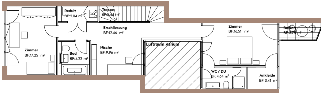
1. Obergeschoss
