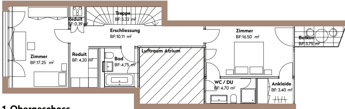
1. Obergeschoss
